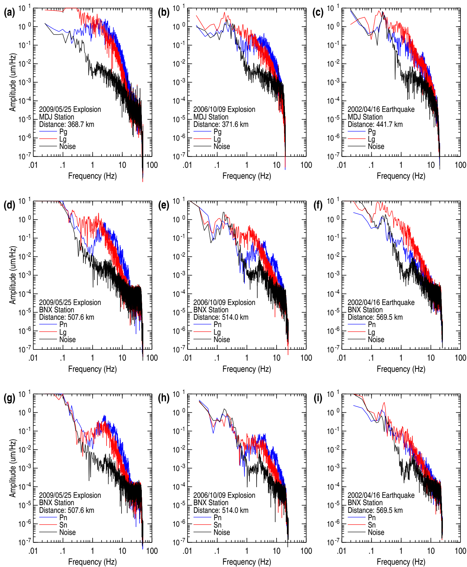
图1 典型的 Pn, Sn, Pg, Lg, 和噪声的谱. 图(a),(d)和(g)为2009/05/25北朝鲜核爆事件;图(b),(e)和(h)为2006/10/09北朝鲜核爆事件;图(c),(f)和(i)为2002/04/16发生在核爆试验点附近的天然地震事件.蓝色线表示P型波,红色线表示S型波,黑色线表示噪声.核爆事件的P波能量较S波能量强,地震事件的S波较P波能量强.
